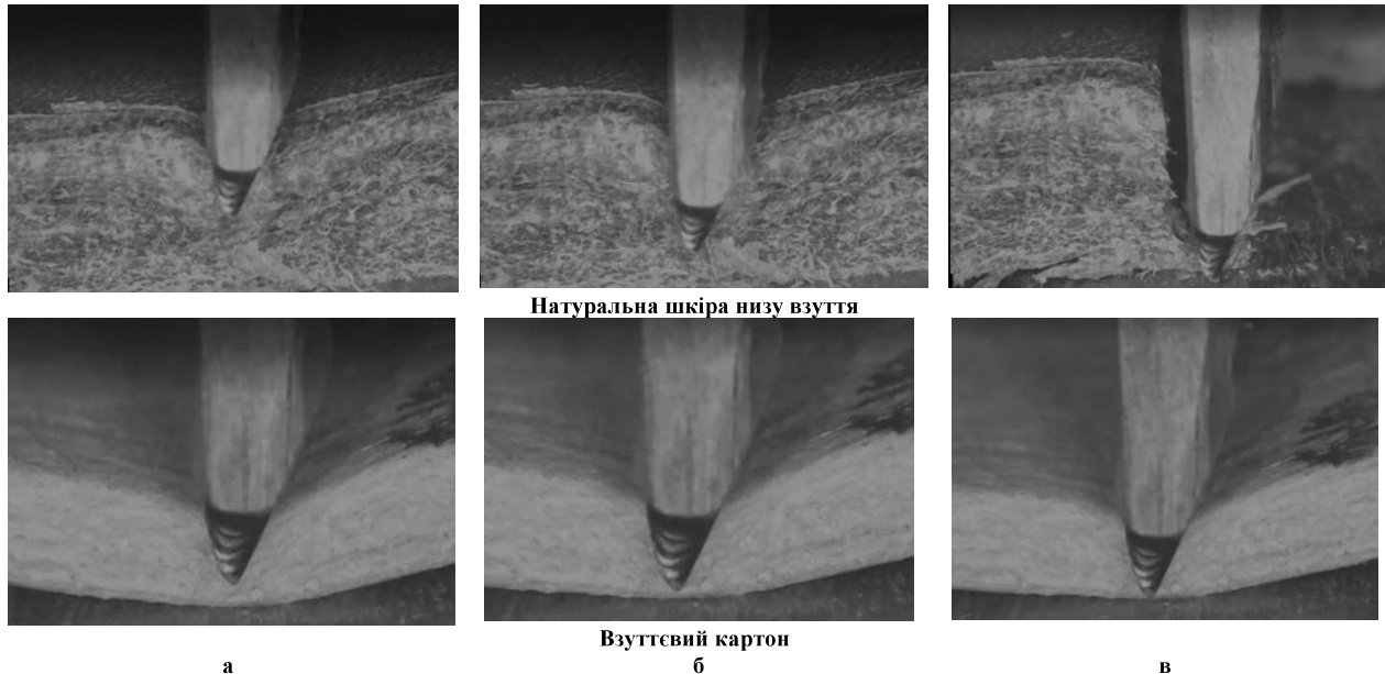
Рис. 5 Етапи занурення різака в матеріал: а – стискання; б – різання; в – розсовування нижнього шару
