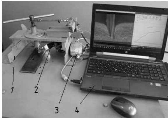
Рис. 1. Установка для дослідження операції вирубування взуттєвих матеріалів в статичному режимі
