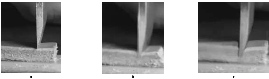
Рис. 9. Етапи занурення різачка в натуральну шкіру низу взуття: а – стиснення; б – різання; в – зона недеформованого матеріалу
