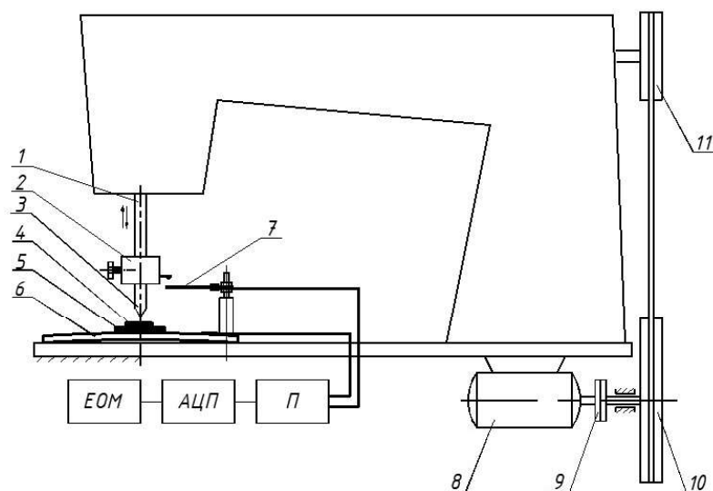
Рис. 6. Експериментальна установка для визначення сили різання в динамічному режимі: 1 – голководій; 2 – тримач; 3 – різак; 4 – матеріал; 5 – вирубна плита; 6 – тензометрична балка для вимірювання сили різання; 7 – тензометрична балка для вимірювання величини занурення різачка в матеріал; 8 – електричний двигун; 9 – муфта; 10 – пасова передача; 11 – махове колесо
